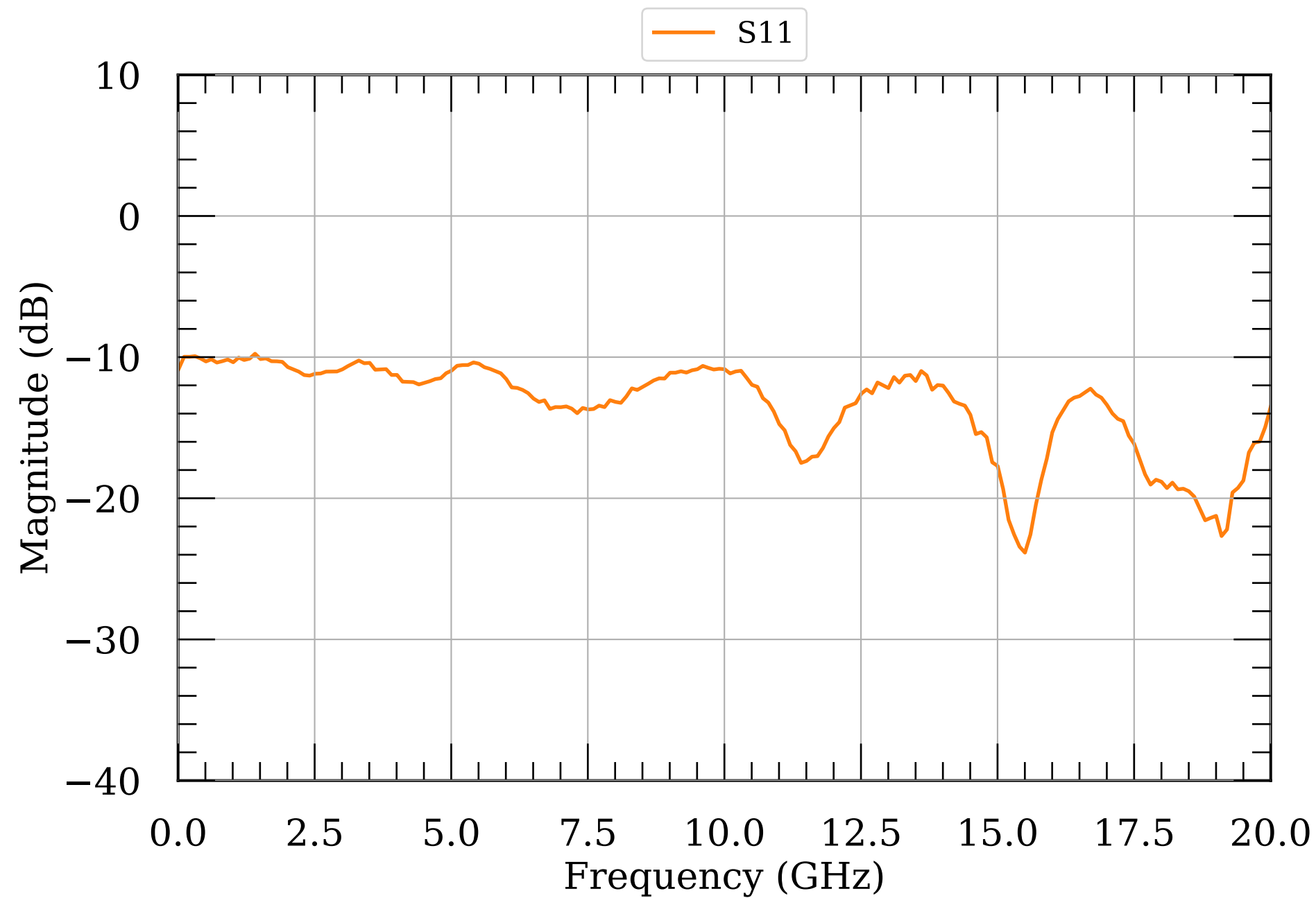
LNA S-params module091
